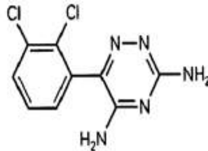
Lamotrigin
