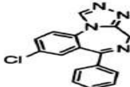
Estazolam
