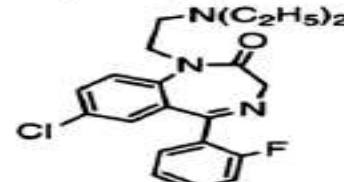
Flurazepam (Dalmane)
