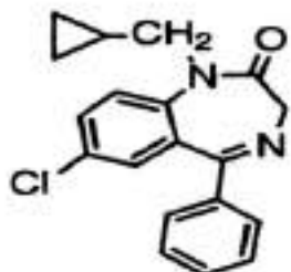
Brazepam
