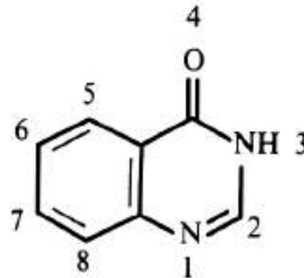
Quinazolone
