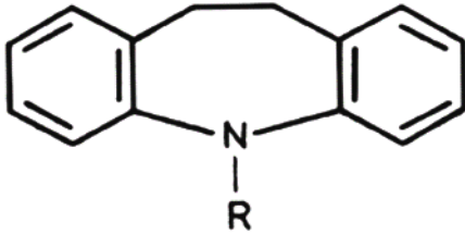
Dibenzo[b,f]azepine
