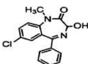
Temazepam
