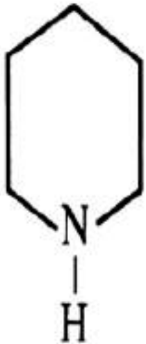
Piperidine
