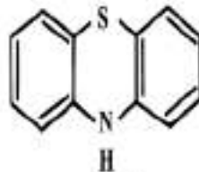
فينوتيازين
