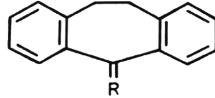
Dibenzo[a,d]cycloheptadiene
