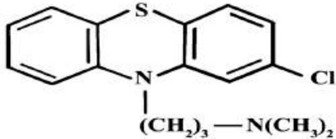
Largactil-Chlorpromazine
